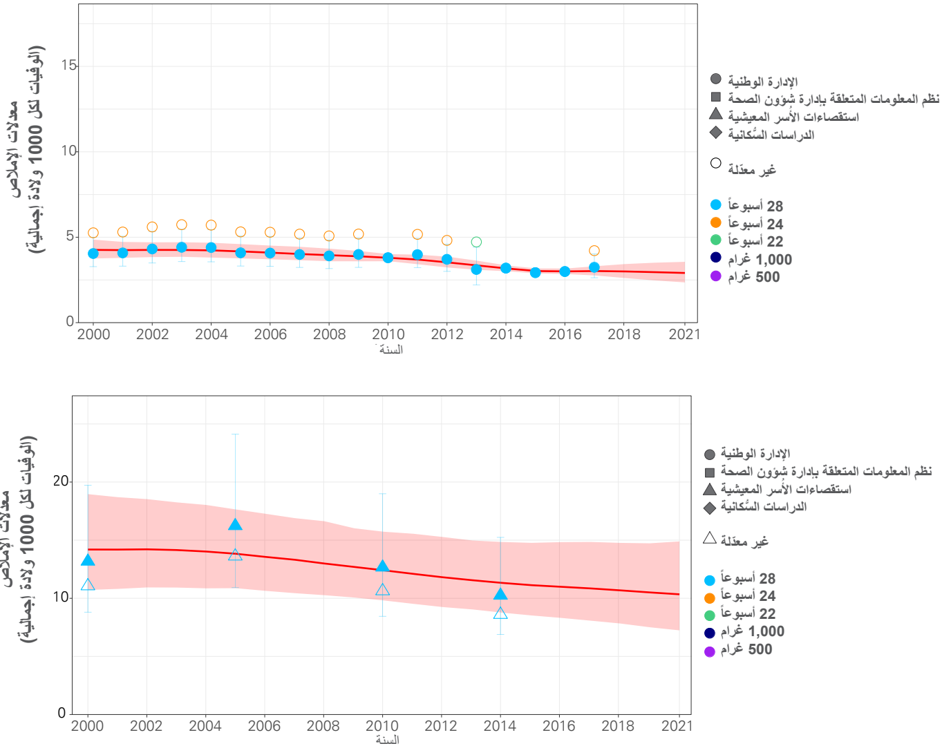
الشكل 4: تقديرات عدم التيقن في البيانات القطرية وتقديرات الاتجاه
