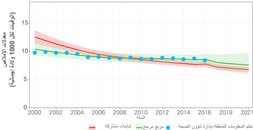
الشكل 3: التباينات المشتركة والبيانات القطرية
